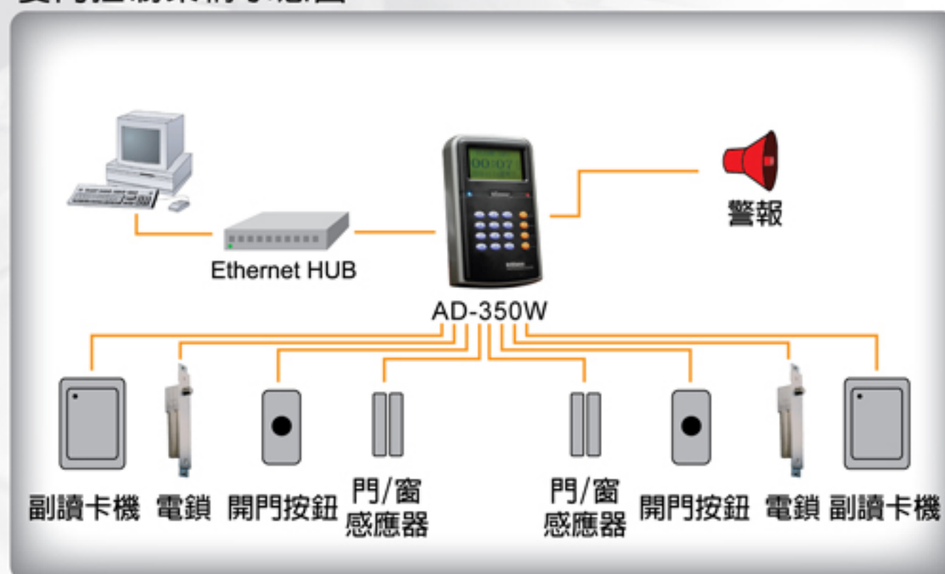
雙門控制架構示意圖
