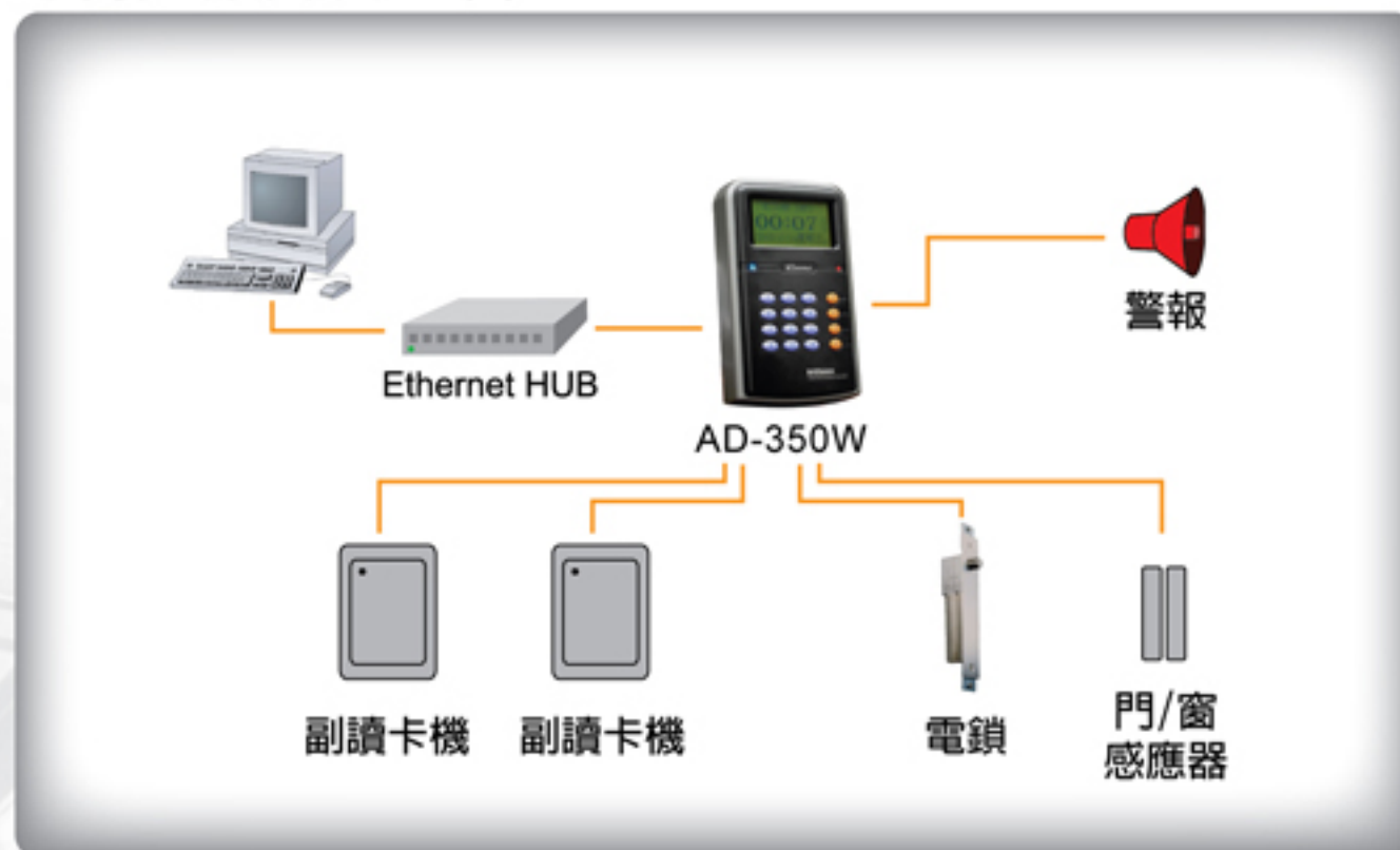
單門控制架構示意圖
